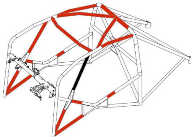
Figure 1 : Emplacements de la garniture d'arceau
